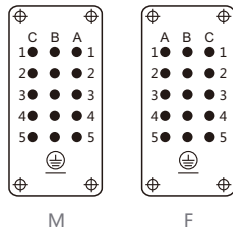
接插针排序
