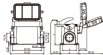
带保护盖
