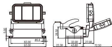
带保护盖
